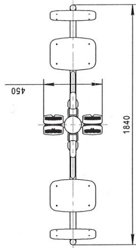
Рисунок 2 - Установка изделия
